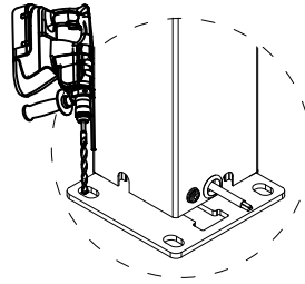
3.12、 Drill bolt holes
